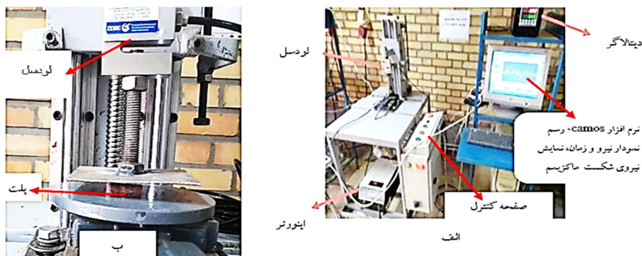
شکل ۳. الف دستگاه آزمون مکانیکی مواد بیولوژیک (ب) نحوه اعمال نیرو در راستای محور افقی پلت
